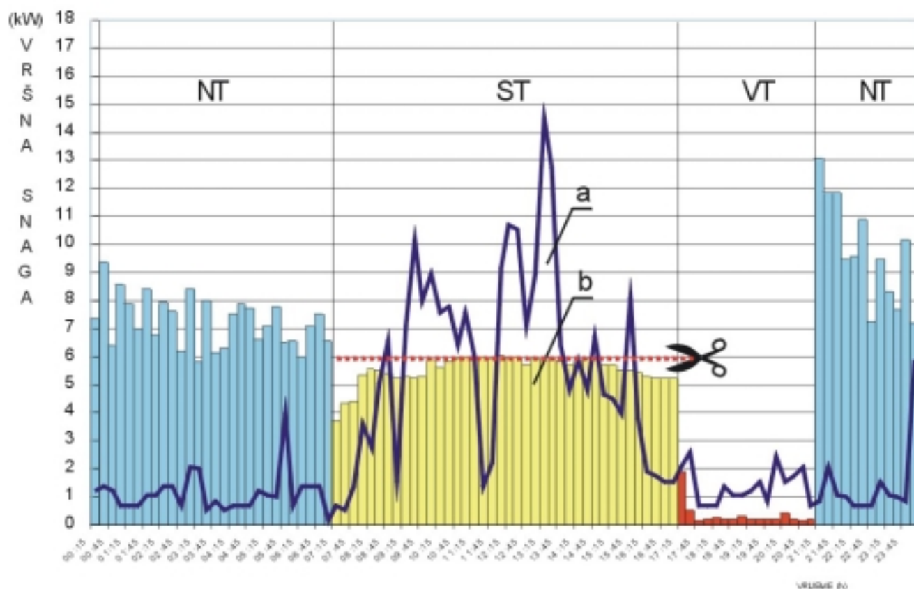
SL.1. KARAKTERISTIČNI DNEVNI DIJAGRAM VRŠNIH SNAGA ZA "MRAMOTERM" - MARINIČI U ZIMSKOM PERIODU :
